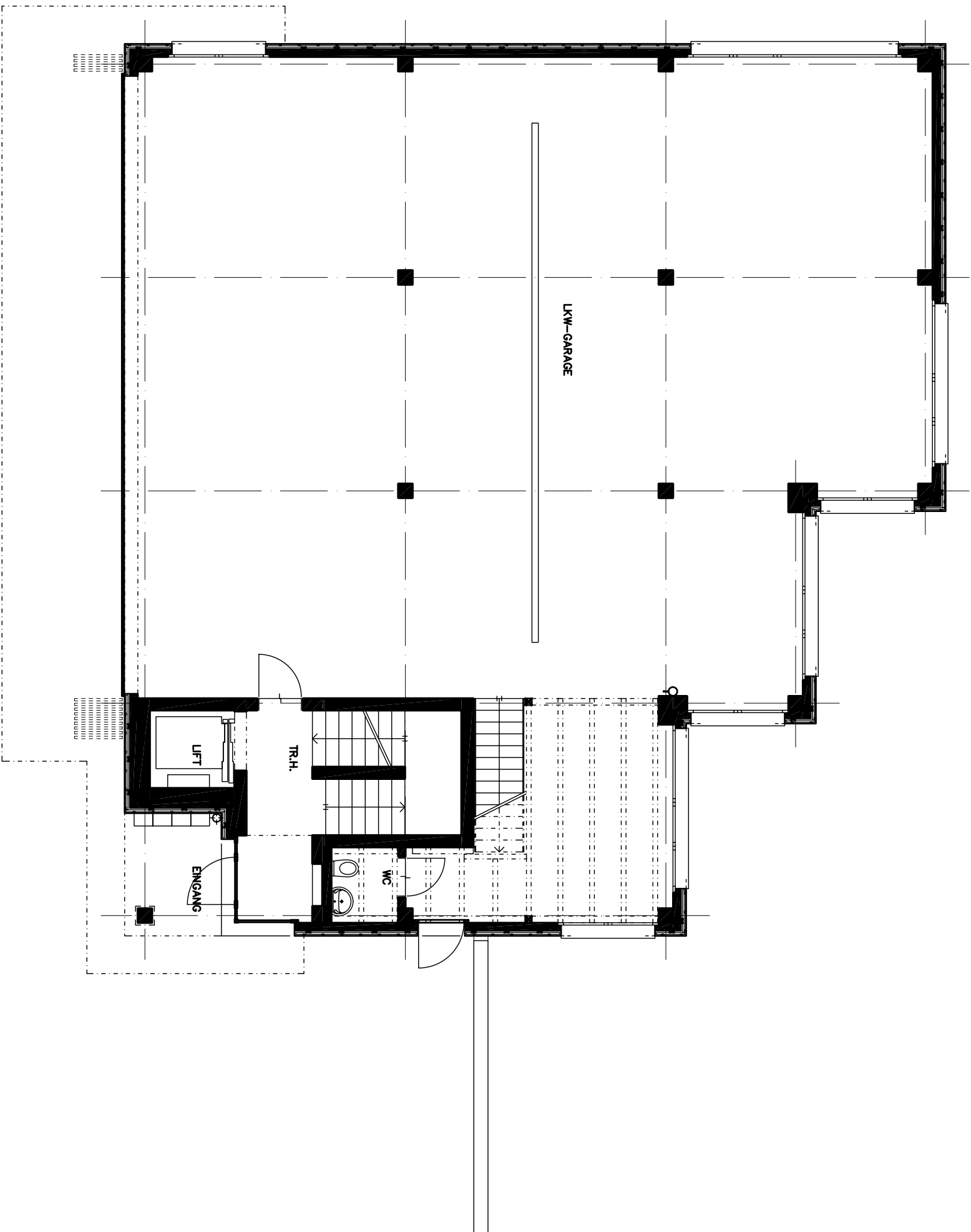
ZWISCHENGESCHOSS EG/1.0G
